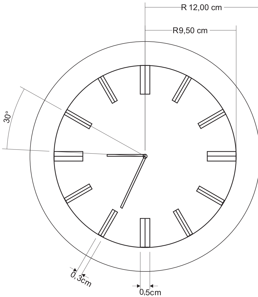
VISTA FRONTAL ESC.: 1:2 EM: CM
